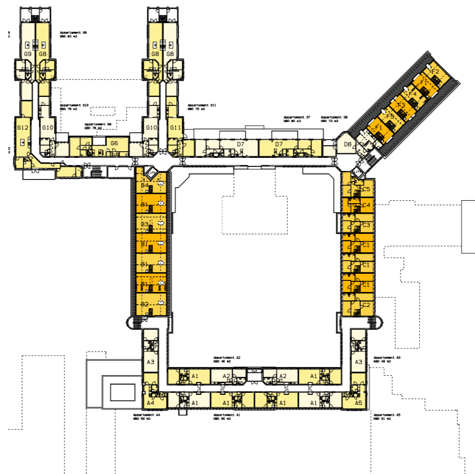
Tweede verdieping
