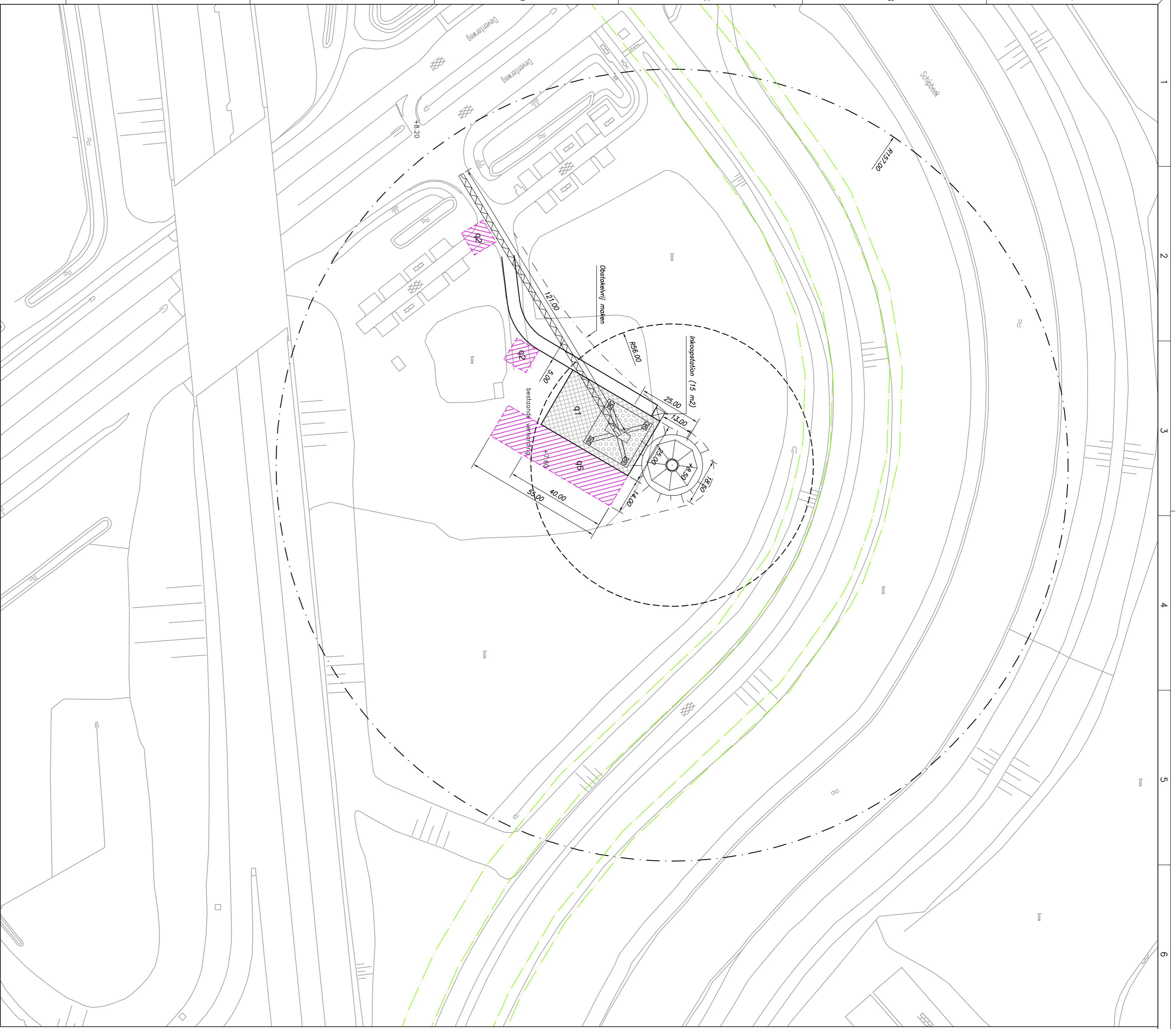
Terrinrichting westelijke windmolen
