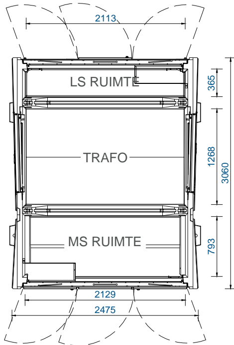
VLOERPLAN
