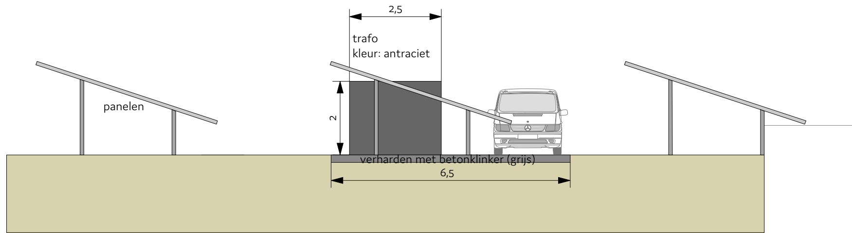
Zijaanzicht trafo
