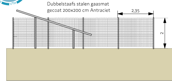
Detail Hekwerk
