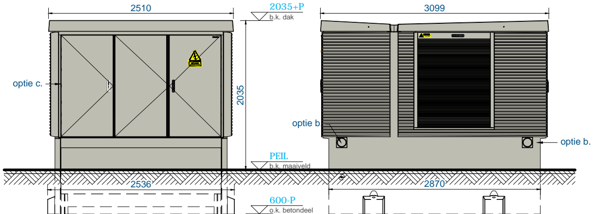
VOORAANZICHT
