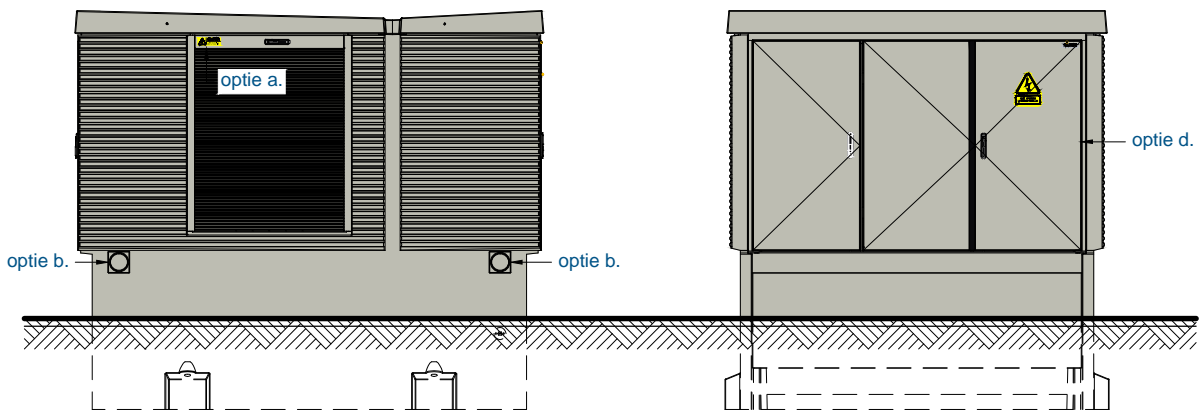
LINKER ZIAANZICHT
